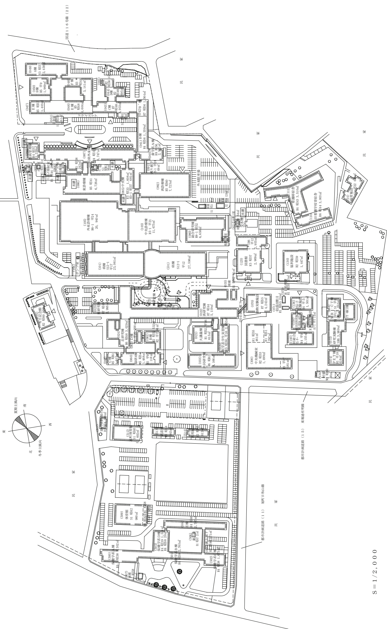
施設配置図
