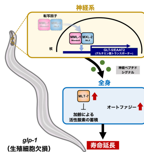
図1. 研究成果概略 神経系の MML-1 は GLT-5 の転写を促進させ、全身レベルでのオートファジー活性化・活性酸素の蓄積抑制をすることで、線虫の寿命を延長させる
