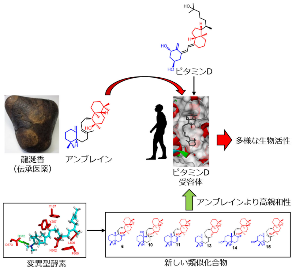
図1：龍涎香の主成分アンブレインのビタミンD受容体結合能発見とアンブレインよりビタミンD受容体に高い親和性を示す化合物の創出
