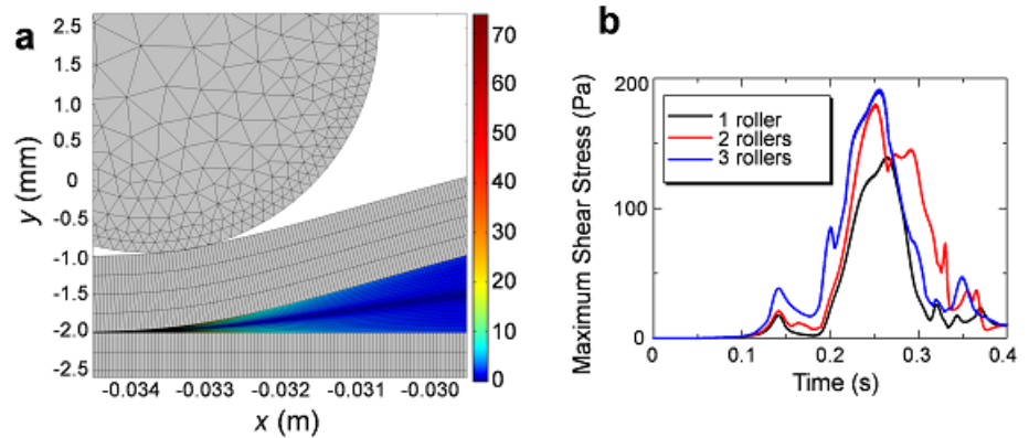
図3 FEM 解析によるペリスタリックポンプのせん断ストレスの評価。 通常の層流に比べて1万倍も高いことが示唆された。
