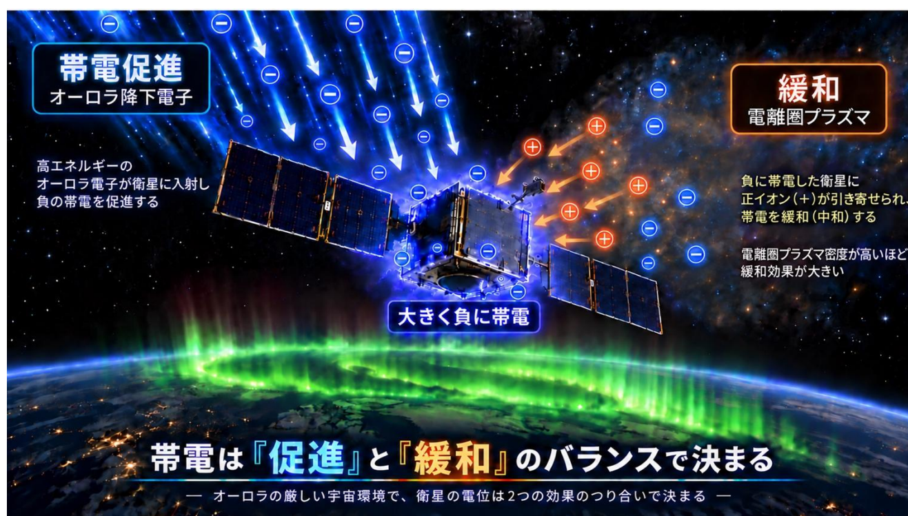
図：本研究で明らかになった人工衛星表面帯電の仕組み。高エネルギーのオーロラ降下電子は衛星の負の帯電を促進し、電離圏プラズマ中の正イオンの流入は帯電を緩和します。衛星の電位は、これらの電流のバランスによって決まります。（本イラストは生成 AI を用いて作成したものです。）
